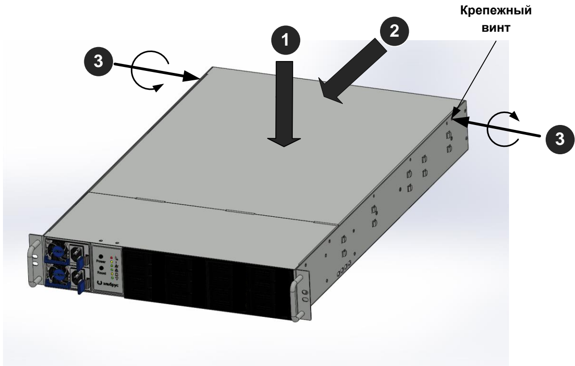
Рисунок 13 – Монтаж крышки корпуса
