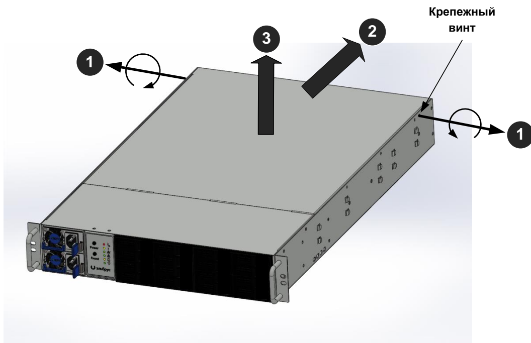
Рисунок 12 – Демонтаж крышки корпуса
