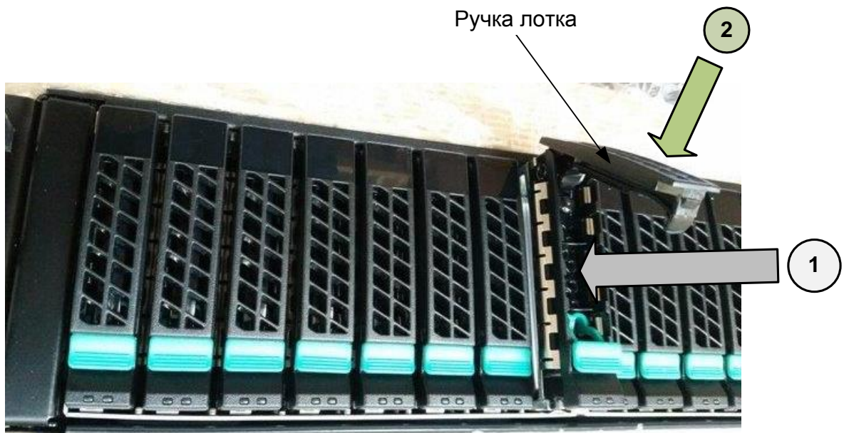
Рисунок 9 – Монтаж накопителя SSD
