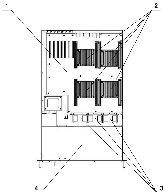
Рисунок 2 – Внешний вид ВП сзади
