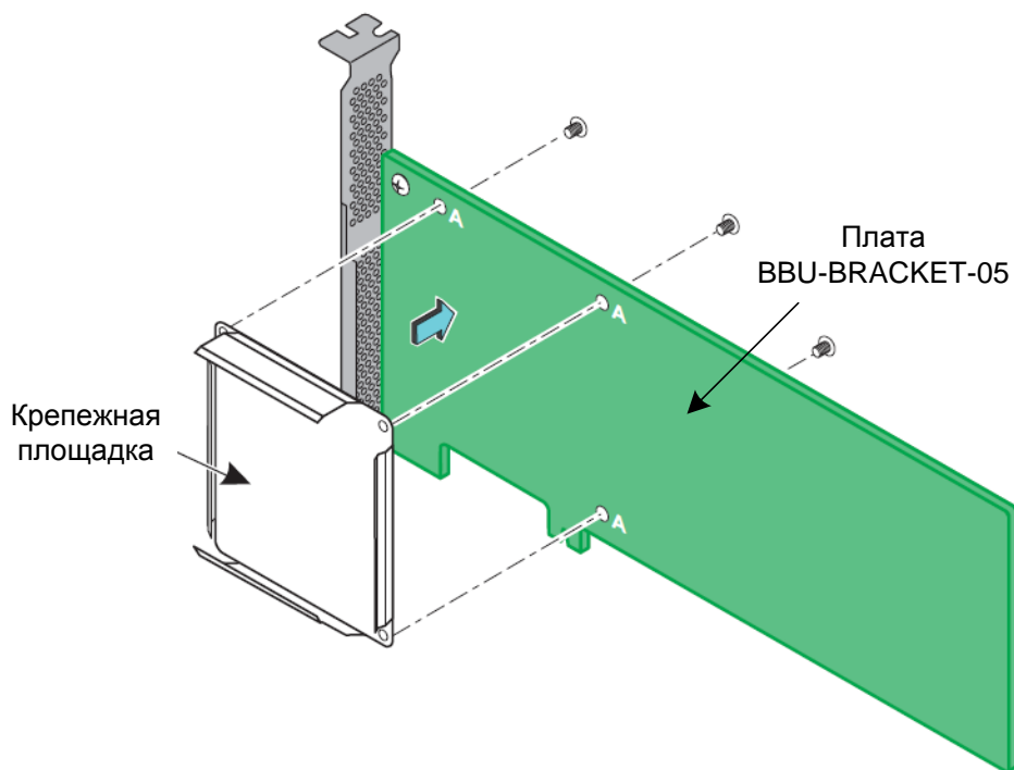
Рисунок 13 - Монтаж крепежной площадки к плате BBU-BRACKET-05
