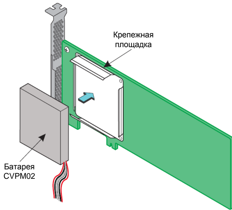
Рисунок 14 - Присоединение батареи CVPM02 к крепежной площадке
