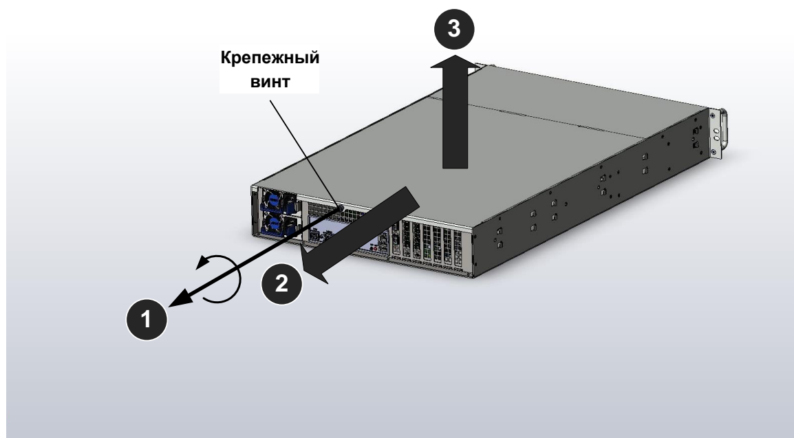
Рисунок 16 – Демонтаж крышки корпуса
