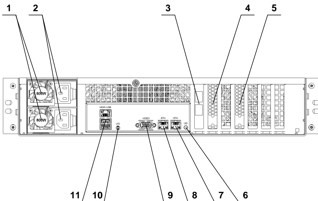
Рисунок 1 – Внешний вид сервера 1Э8-2U спереди
